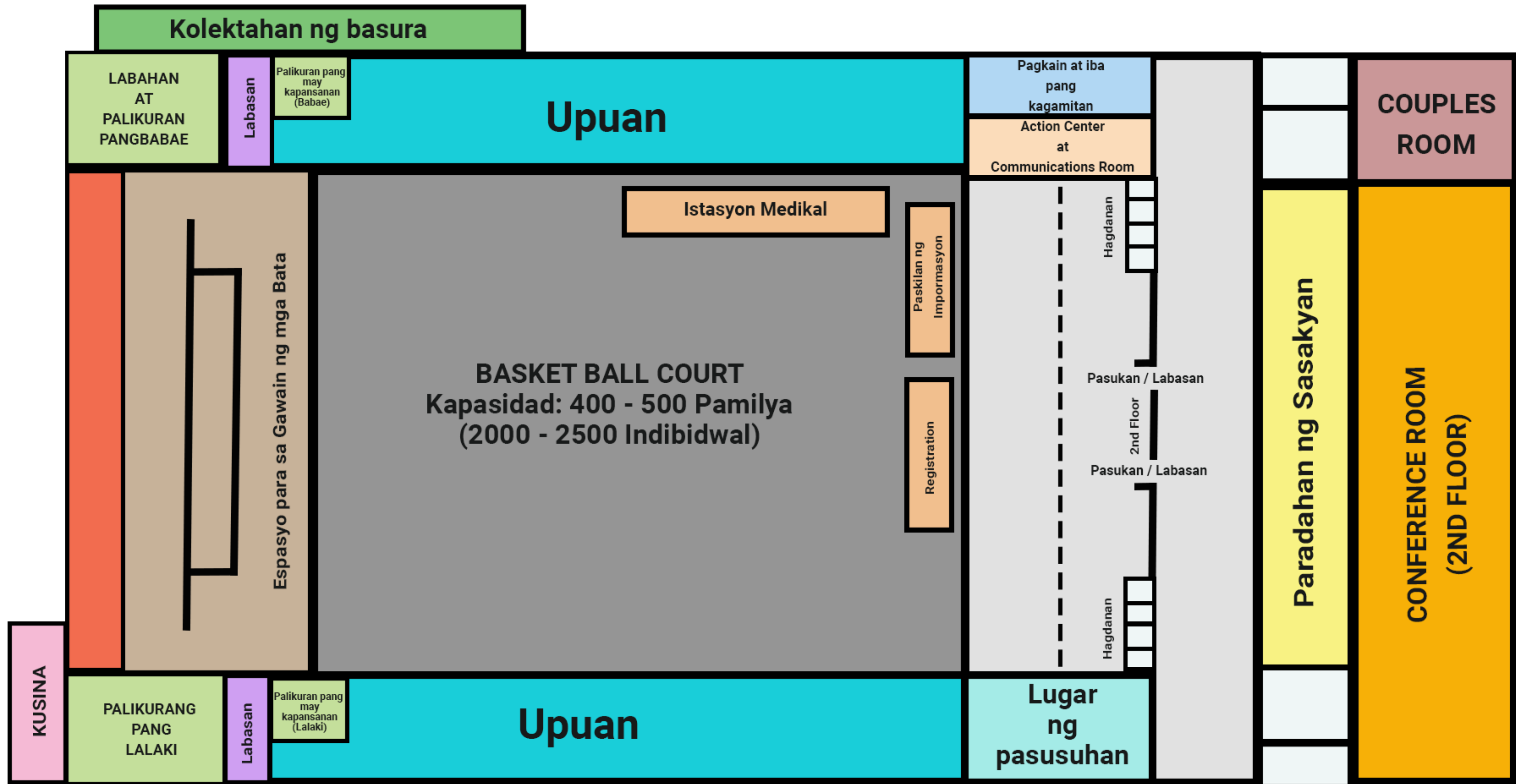
PLANO PARA SA EVACUATION CENTER GMACC
